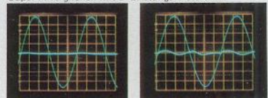
Wellenformen und Spektren der Verzerrung: Super-A verglichen mit B-Leistungsverstärkern
