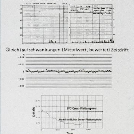
Geräuschspannungsabstand und Gleichlaufschwankungen Rumpelgeräuschspannungsabstand (IEC-B)
